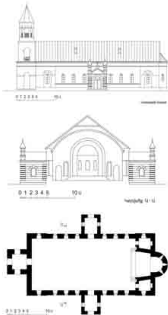
Ախալցխա. Սբ. Ամենափրկիչ եկեղեցու հարավային ճակատը, կտրվածք դեպի արևելք և հատակագիծը (չափ.՝ Ալեքսանդր Իգիթյանյանի, հրատարակության պատրաստող՝ Աշոտ Չակոբյան)
