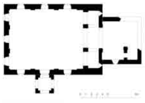
Ախալցխա. Երևման Սբ. Խաչ եկեղեցու հատակագիծը
