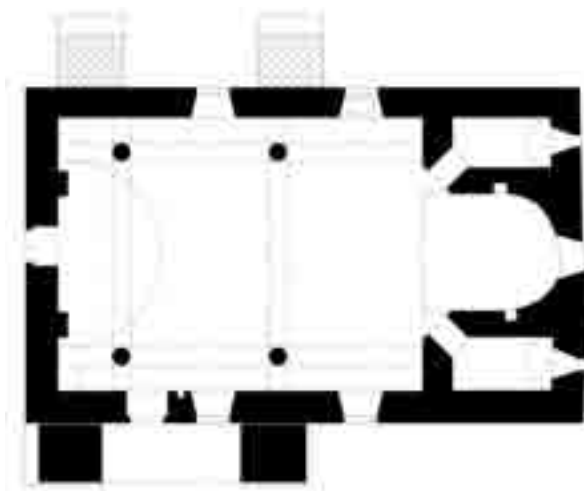
Նաղխրեր. Սբ. Փրկիչ եկեղեցու ներքին տեսքը դեպի արևելք, հատակագիծը (չափ.՝ Ա. Դակոբյանի) և բանալին (լուս.՝ 2007 թ.)
