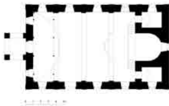
Պամաճ Մեծ (Վարի Պամաճ). Սբ. Խաչ եկեղեցու հատակագիծը (չափ.՝ Ա. Դակոբյանի, 2007 թ.)
