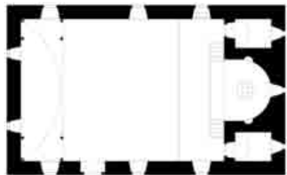
Ծուղորութ. Սբ. Սիոն եկեղեցու հարավային ճակատից բացված միակ մուտքի փայտակերտ դուռը (ուս.՝ 1988 թ.) և հատակագիծը (չափ.՝ Ա. Գակոբյանի, 2007 թ.)
