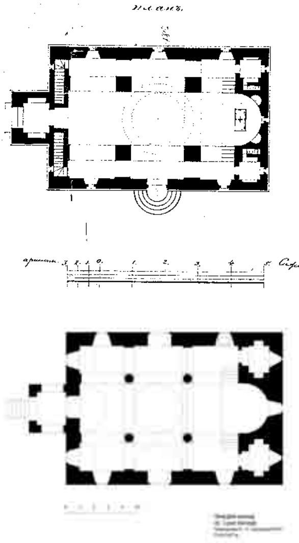
Ախալցխա. Սբ. Վարդանանց եկեղեցու հատակագծերն ըստ մասագծի (1861 թ.) և ըստ իրական կառույցի (չափ.՝ Ա. Դակոբյանի)
