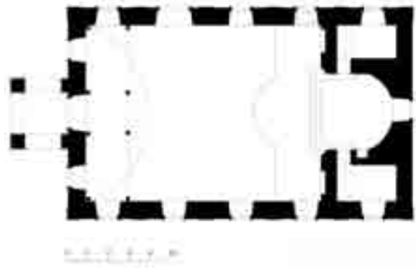
ԾԻՆՈՒԲԱՆ. Սբ. Աստվածամայր եկեղեցու հյուսիսային կողմում եկեղեցաձև տապանաքարով հավերժացված հոգևորականների շիրմներ և եկեղեցու հատակագիծը (չափ.՝ Ա. Չակոբյանի)
