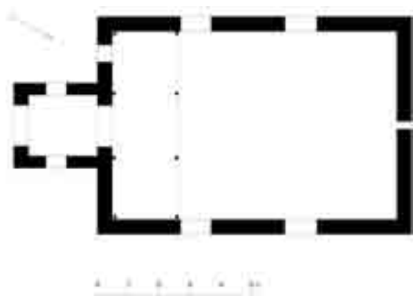
Ղուլալիս. Սբ. Խաչ եկեղեցու տեսքը հարավ-արևելքից, շինարարական արձանագրությունը (ուս.՝ 2007 թ.) և հատակագիծը (չափ.՝ Ա. Գակոբյանի)
