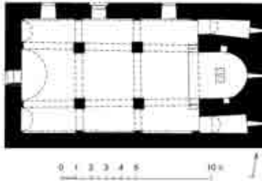
Սբ. Խաչ եկեղեցու հատակագիծը (չափ.՝ Ա. Հակոբյանի, 2018 թ.)
