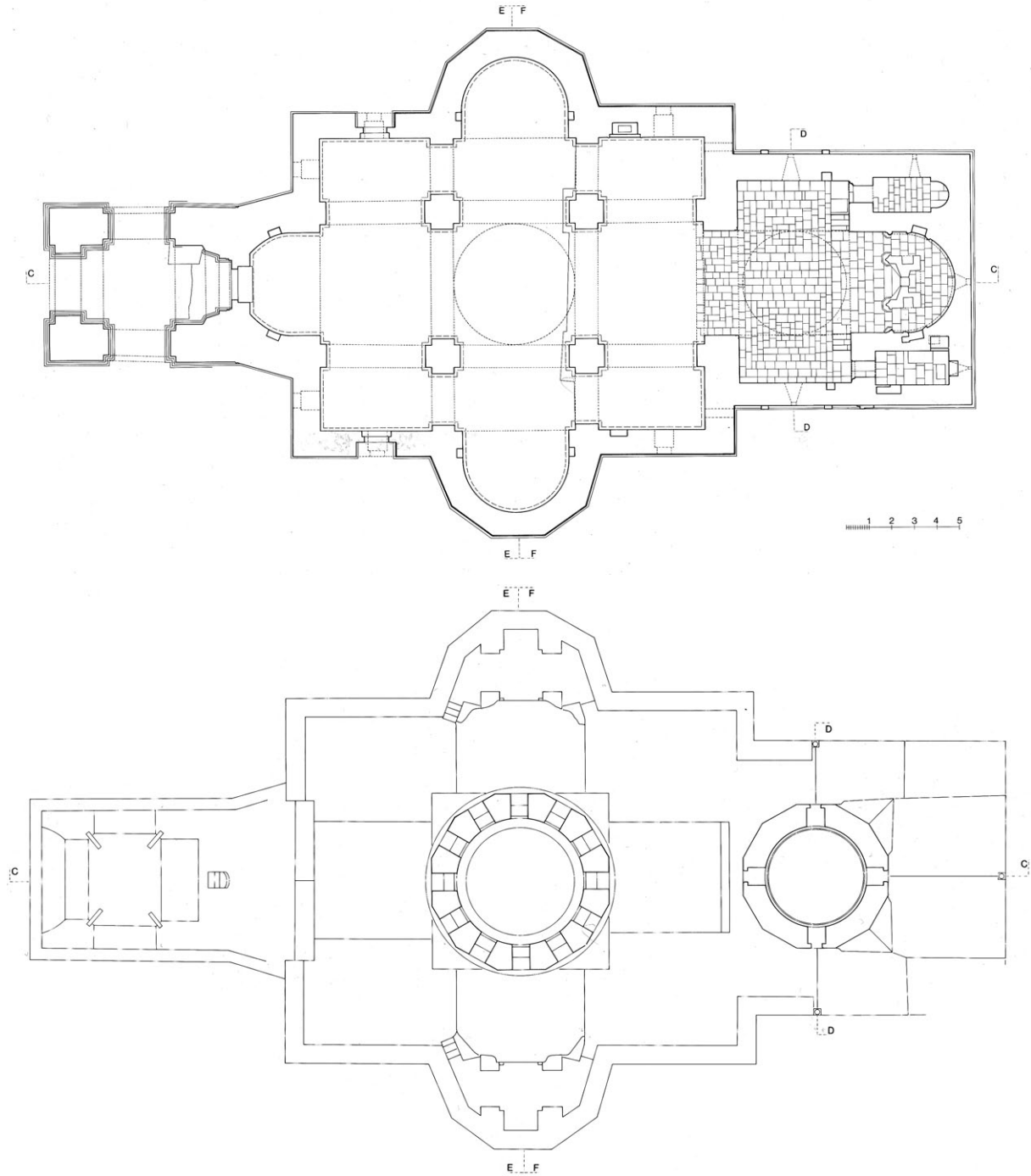
Թադեոս առաքյալի վանք. գավիթ-եկեղեցու և եկեղեցու կտրվածքները դեպի արևելք և դեպի արևմուտք (չափ.՝ ծարտ. դր. Արմեն Գախնազարյանի, 1968 թ.)
