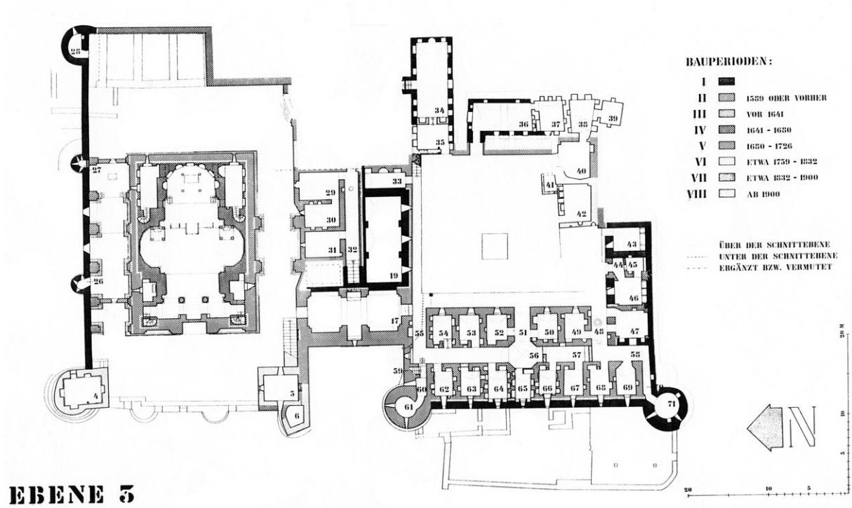
Մաղարդա Սբ. Ստեփանոս ճախավկայի վանքի գլխավոր հատակագիծը (չափ.՝ ճարտ. դր. Գաբրիելոտ Գոֆրիխտերի)
