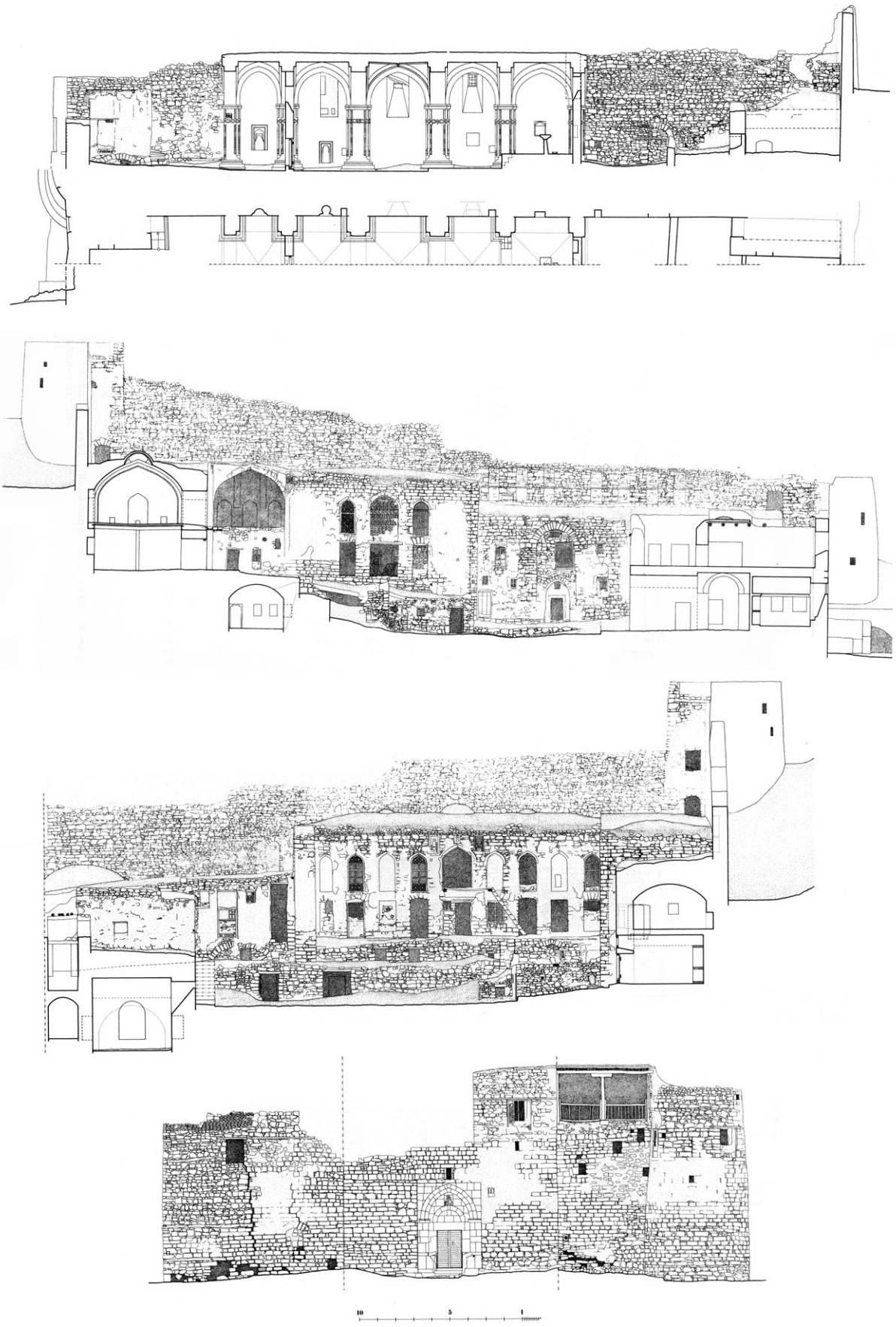
Մաղարդա Սբ. Ստեփանոս նախավկայի վանքի շրջապարսպի և օժանդակ շինությունների ճակատները դեպի հյուսիս, հարավ, արևելք և արևմուտք (չափ.՝ ճարտ. դր. Գարթեմուտ Գոֆրիխտերի)
