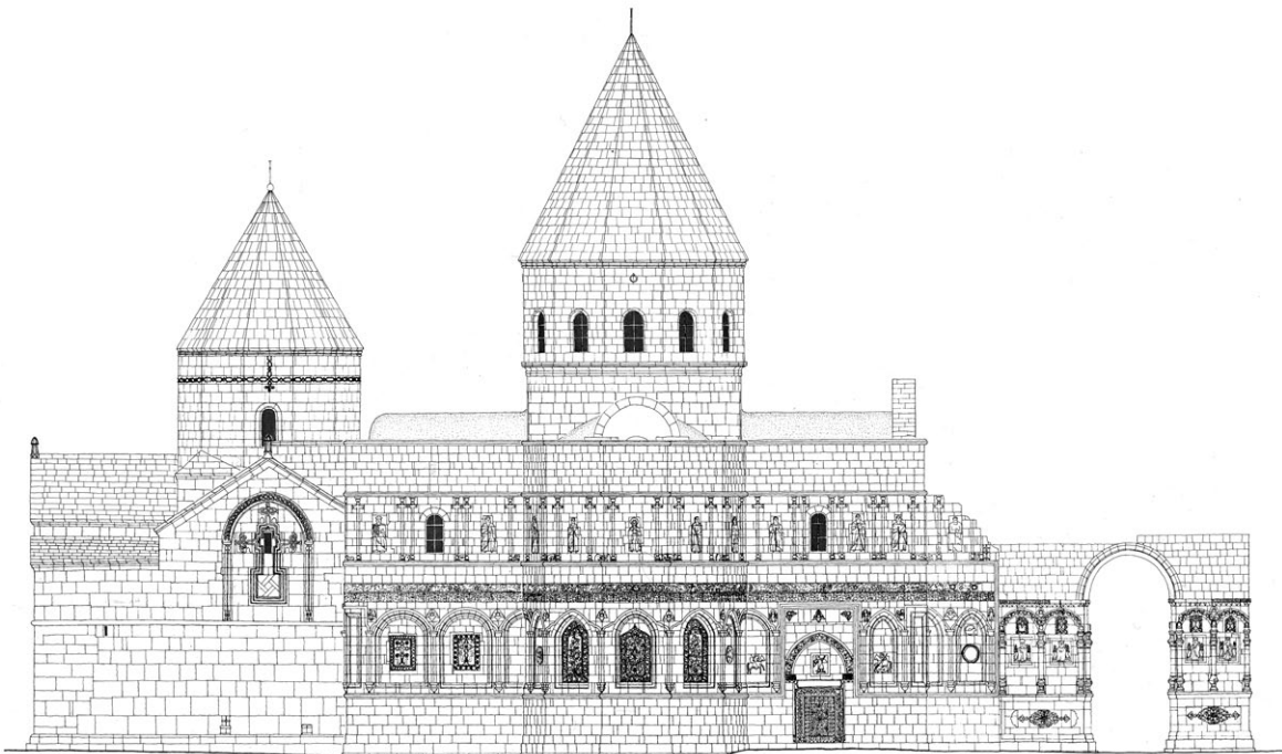
Թադեոս առաքյալի վանք. եկեղեցու, գավիթ-եկեղեցու և զանգակատան հարավային և հյուսիսային ճակատները (չափ.՝ ճարտ. դր. Արմեն Չախնազարյանի, 1968 թ.)
