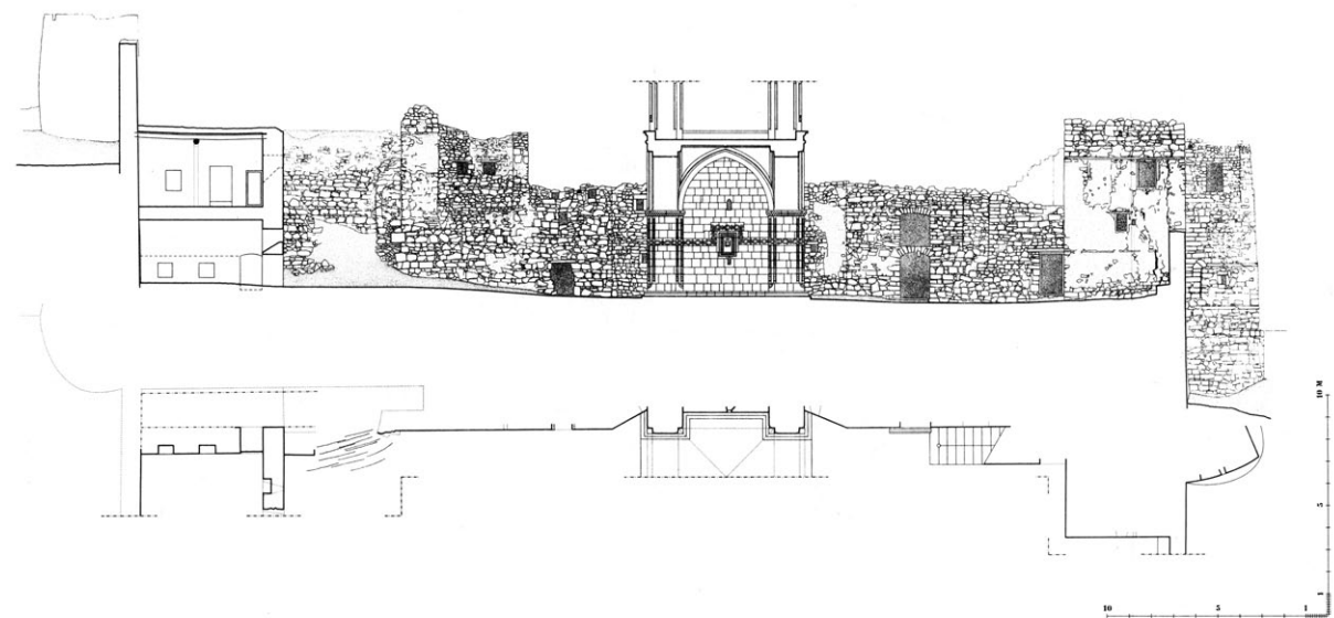
Մաղարդա Սբ. Ստեփանոս նախավկայի վանքի լայնակի կտրվածքները դեպի հյուսիս, արևելք և հարավ (չափ.՝ ճարտ. դր. Հարթմուտ Դոֆրիլտերի)
