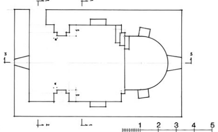
Սբ. Սանդուխտ մատուռի հատակագիծը (չափ.՝ ճարտ. դր. Արմեն Հախնազարյանի)
