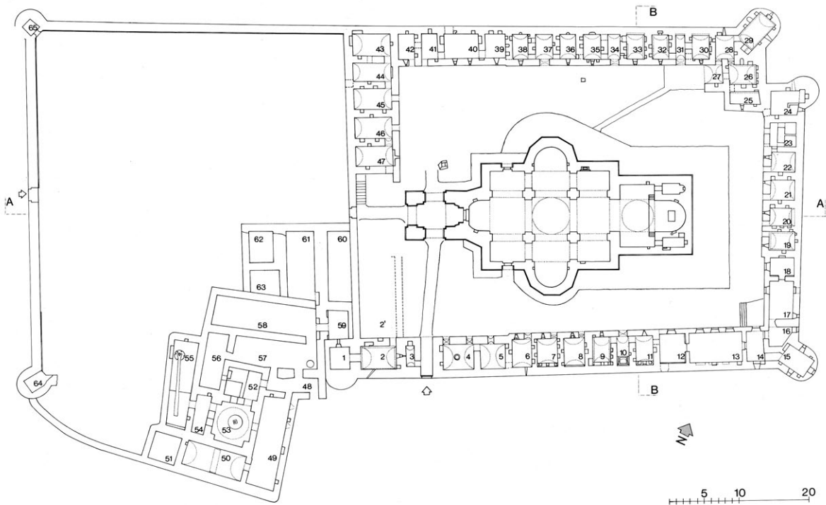
Թադեոս առաքյալի վանք. համալիրի գլխավոր հատակագիծը (չափ.՝ ճարտ. դր. Արմեն Չախնազարյանի, 1968 թ.)
