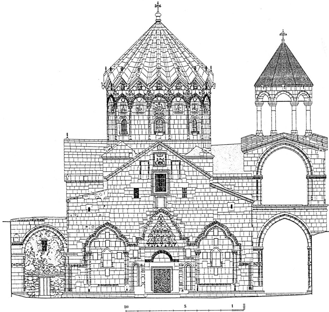
Մաղարդա Սբ. Ստեփանոս նախավկայի վանքի եկեղեցիների և զանգակատան արևմտյան ճակատը (չափ.՝ ճարտ. դր. Գարթմուտ Գոֆրիխտերի)
