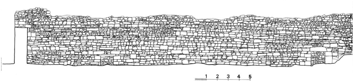
Թադեոս առաքյալի վանք. շրջապարսպի հարավային ճակատը, հյուսիսային պարսպապատի կենտրոնական հատվածը և արևմտյան պարսպի հյուսիսային հատվածն արտաքին բակի կողմից
