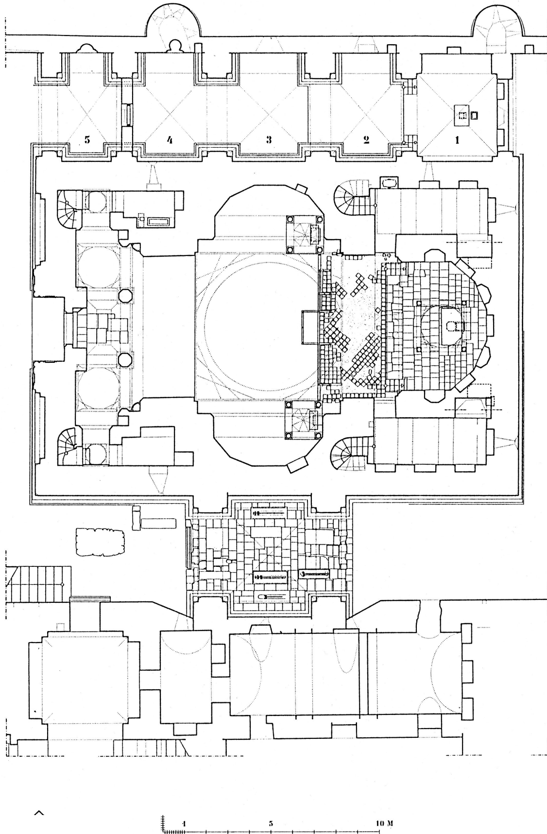
Մաղարդա Սբ. Ստեփանոս ճախավայրի վանքի զույգ եկեղեցիների և հարակից կառույցների հատակագիծը (չափ.՝ ճարտ. դր. Գարթմուտ Դոֆրիստերի)
