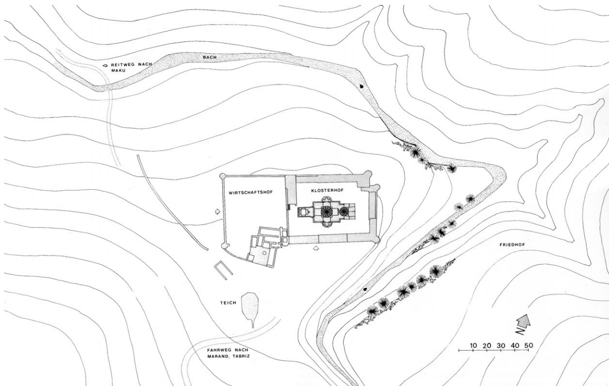
Թադեոս առաքյալի վանք. տեղանքի համույթը (չափ.՝ ճարտ. դր. Արմեն Չախնազարյանի, 1968 թ.)
