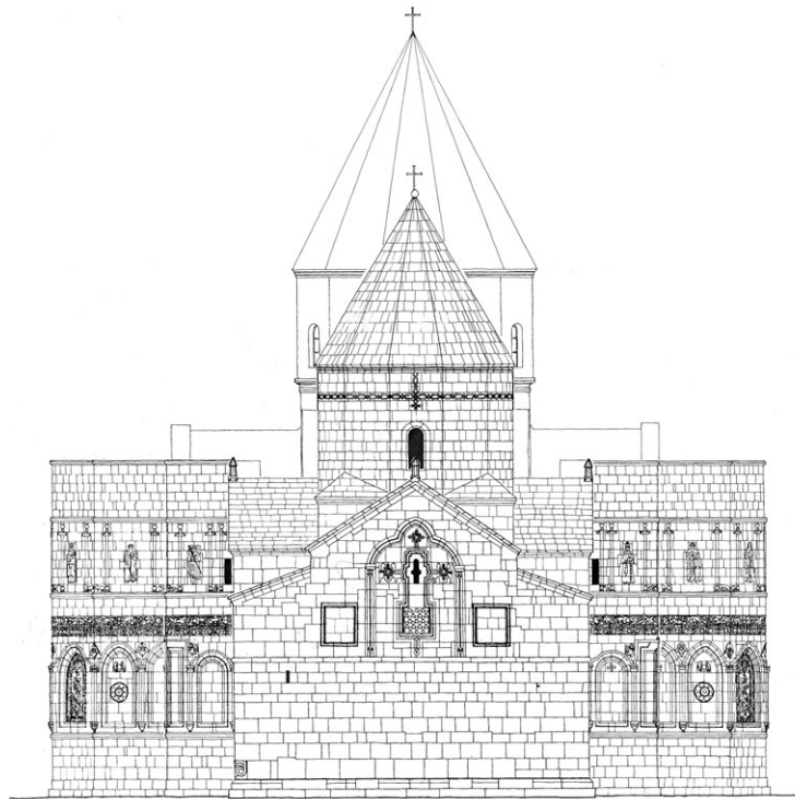
Թադեոս առաքյալի վանք. կենտրոնական կառույցների արևմտյան և արևելյան ճակատները (չափ.՝ ճարտ. դր. Արմեն Հախնազարյանի, 1968 թ.)
