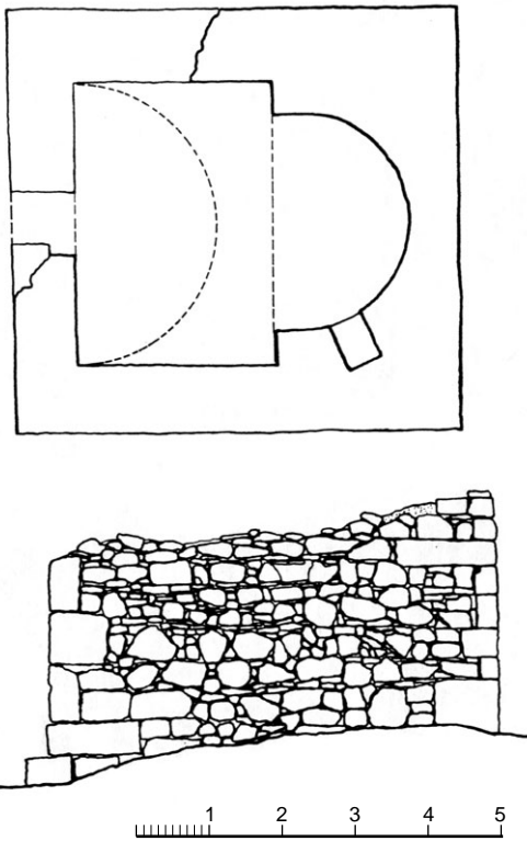
Սք. Աստվածածին կամ Նահատակության տեղի փոքր մատուռի հատակագիծն ու հարավային ճակատը (չափ.՝ ճարտ. դր. Արմեն Դախնազարյանի)
