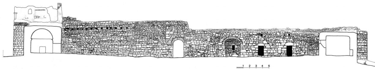
Թադեոս առաքյալի վանք. հյուսիսային, հարավային, արևելյան և արևմտյան պարիսպներից կից օժանդակ կառույցների ճակատները բակի կողմից
