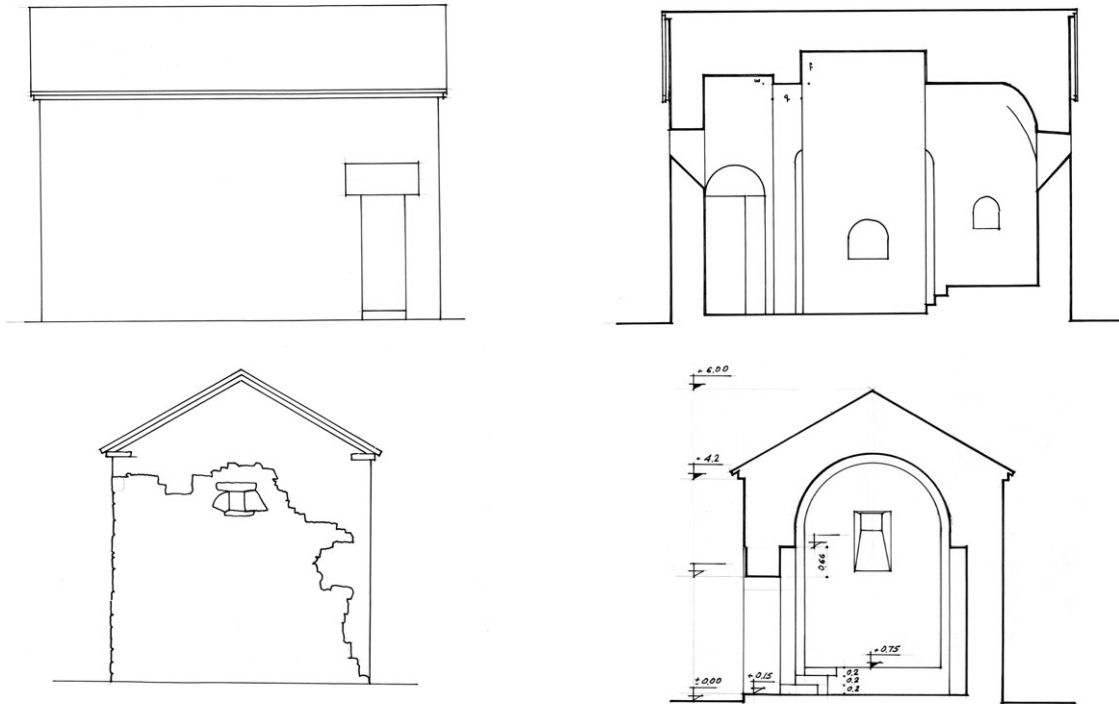
Սբ. Սանդղոխտ մատուռի հարավային և արևմտյան ճակատները և կտրվածքները դեպի հյուսիս և արևելք (չափ.՝ ճարտ. դր. Արմեն Գախաբյանի)
