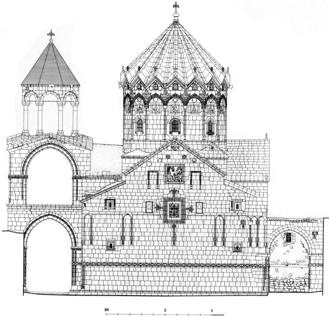
Մաղարդա Սբ. Ստեփանոս նախավկայի վանքի եկեղեցիների և զանգակատան արևելյան ճակատը (չափ.՝ ճարտ. դր. Հարթմուտ Հոֆրիխտերի)
