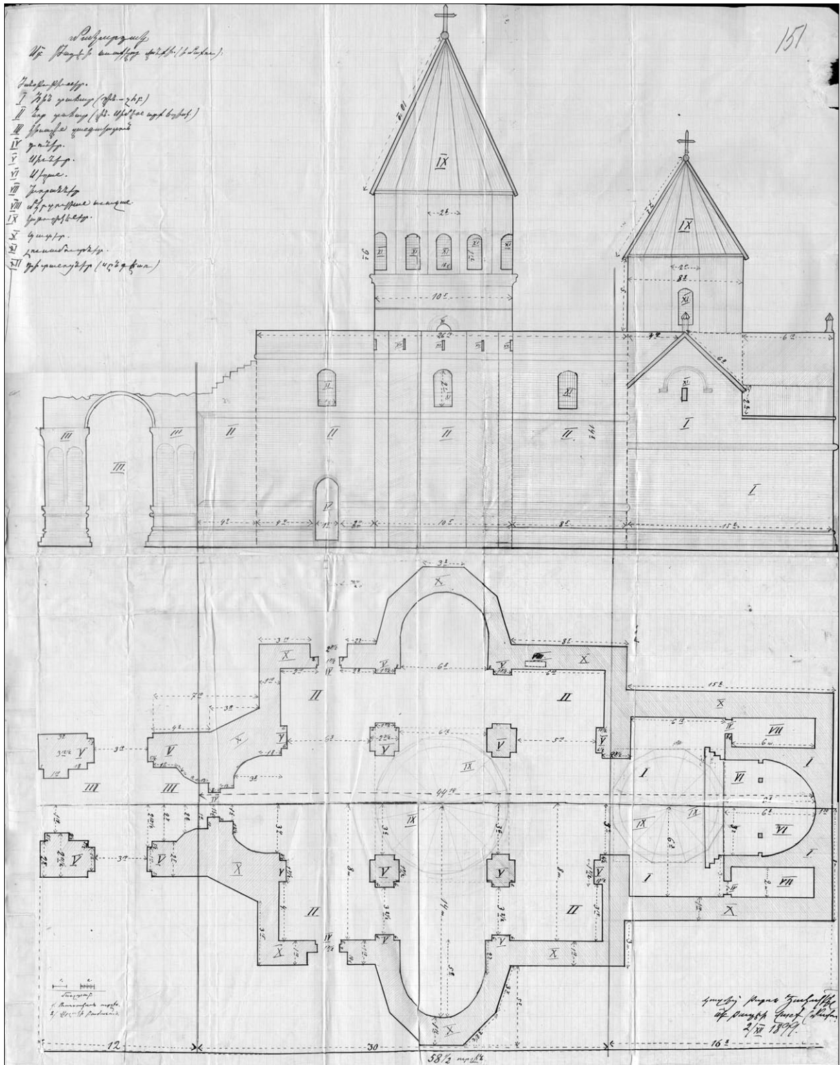
Թաղեոս առաքյալի վանք (չափ.՝ ճարտ. Թաթոս Հակոբյանի, 1899 թ.)
