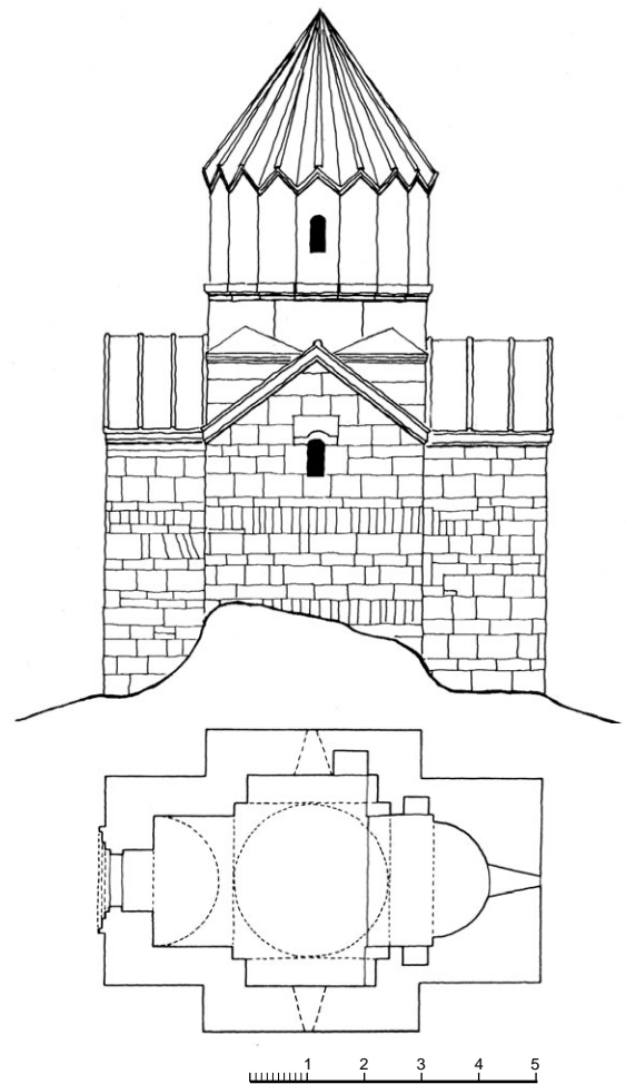
Ծործորի վանքի եկեղեցին նոր վայրում վերականգնելու ընթացքում, հատակագիծն ու հյուսիսային ճակատը
