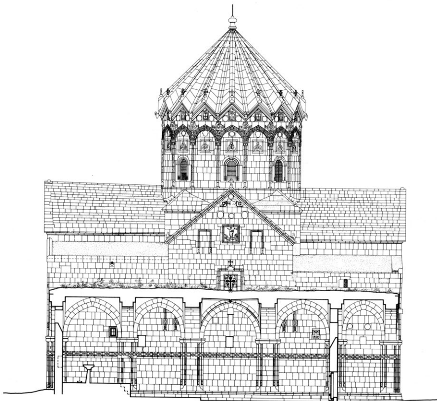
Մաղարդականքի Սբ. Ստեփանոս եկեղեցու հարավային և հյուսիսային ճակատները (չափ.՝ ճարտ. դր. Գարթմուտ Գոֆրիխտերի)
