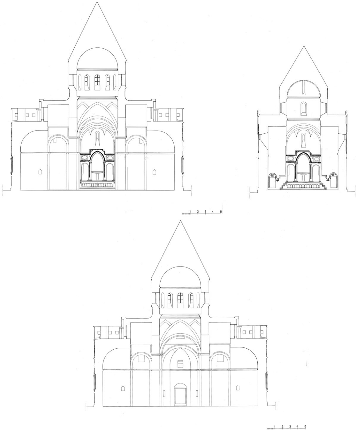
Թադեոս առաքյալի վանք. գավիթ-եկեղեցու և եկեղեցու կտրվածքները դեպի արևելք և դեպի արևմուտք (չափ.՝ ճարտ. դր. Արմեն Գախճազարյանի, 1968 թ.)
