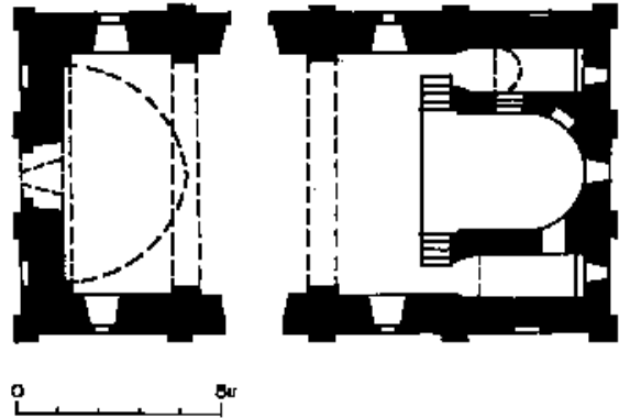
ՄՂՆԱԽ. Սր. Գևորգ եկեղեցու հասակագիծը
