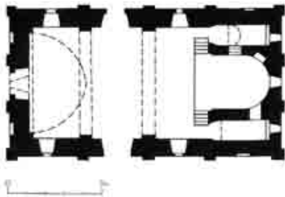
ՈՐՐԻԱԹՈՒԲԱՆ. Սր. Սարգիս եկեղեցու հատակագիծը
