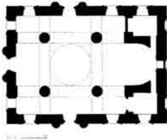
ՉԱՔԱԹԱՍԱ. Սբ. Գևորգ եկեղեցու հասակագիծը
