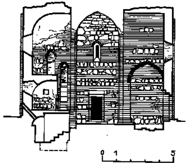
ԳՐԵՄ. Սր. Աստվածածին եկեղեցու կտրվածքը դեպի արևելք և հարավ
