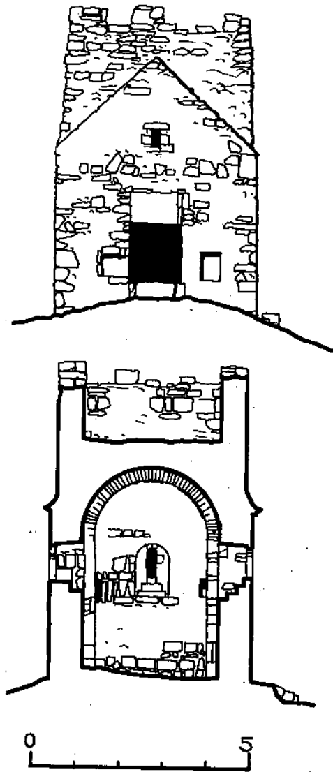
ԳՐԵՄ. «Աշտարակավոր» եկեղեցու տեսքը արևմուտքից և հարավ-արևմուտքից: Նույն եկեղեցու հատակագիծը, արևմտյան ճակատը և կտրվածքները դեպի հարավ և
