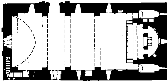
ԹԵԼԱՎ. ՉՎԵԼԳԱԼԱՎԱՆԻ ՍՐ. ԳԵՎՈՐԳ ԵԿԵՂԵՑՈՒ ՀԱՍՏԱԿԱԳԻԾ
