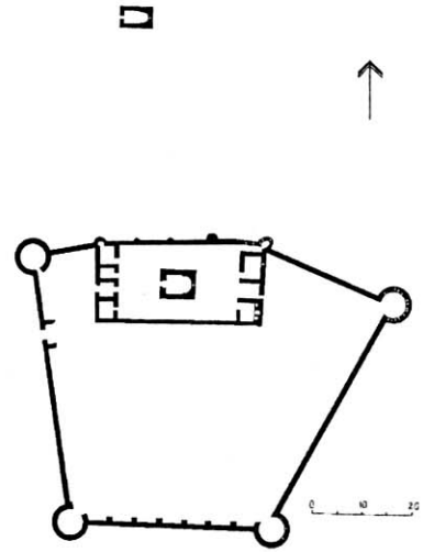
Բնիճորի Մեծ վանքի հատակագիծը
