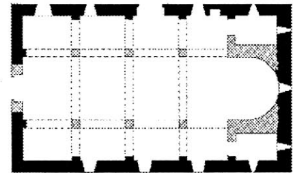
Սբ. Աստվածածին եկեղեցու հատակագիծը
