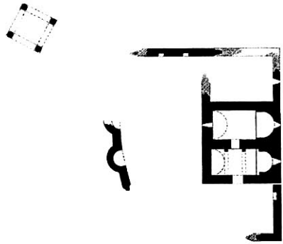
Սք. Կիրակի հուշարձանախմբի հատակագիծը
