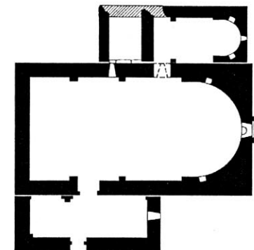
Բնիձորի Միջին վանքի հատակագիծը
