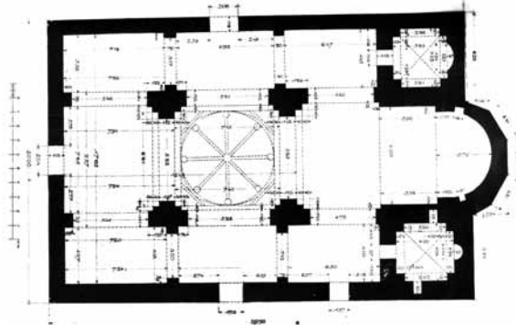
Մրեն. Կաթողիկե եկեղեցու հատակագիծն ըստ Թ. Թորամանյանի
