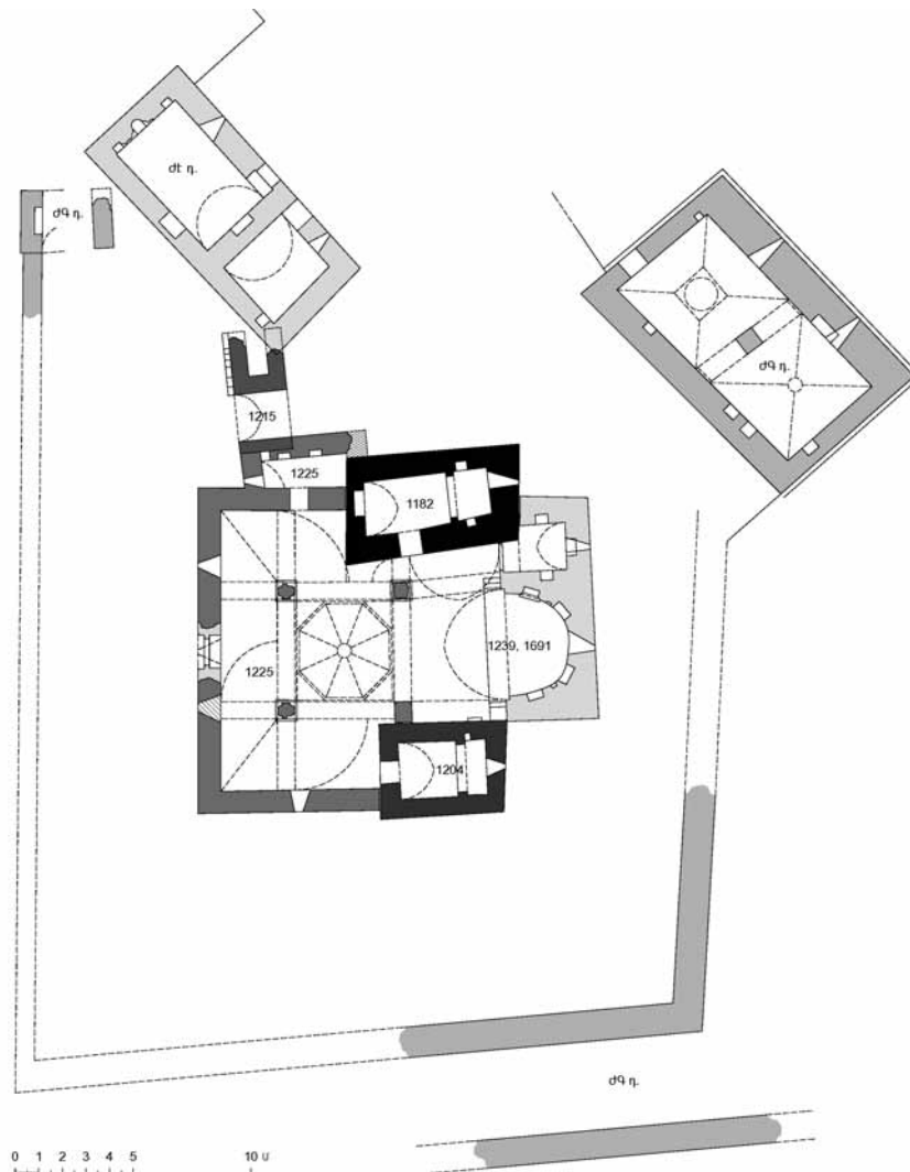
Խաթրավանքի գլխավոր հատակագիծը (չափ.՝ Է. Աբրահամյանի և Ս. Կարապետյանի, 2005 թ., հրատ. պատրաստեց Ճարտ. Ա. Հակոբյանը, 2012 թ.)
