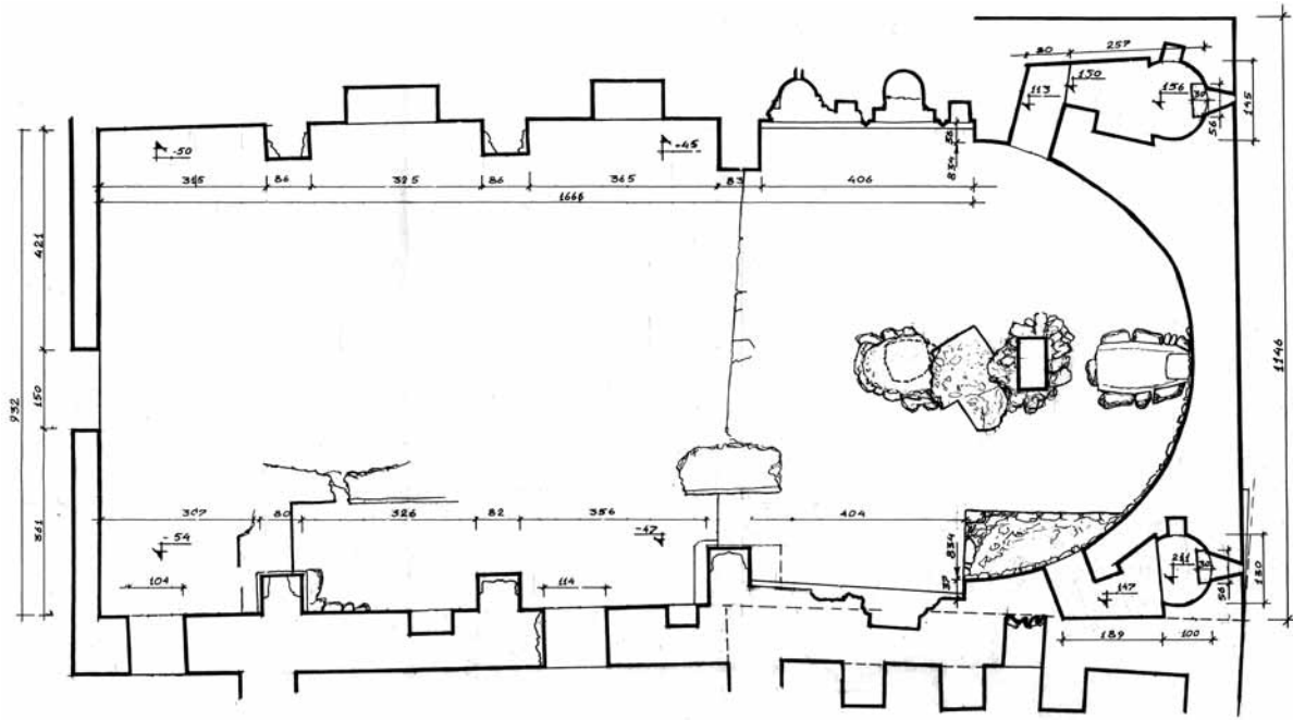
Աբ. Դաղի եկեղեցու հատակագիծը պեղումներից հետո (չափ.՝ Ս. Այվազյանի, 2008 թ.)
