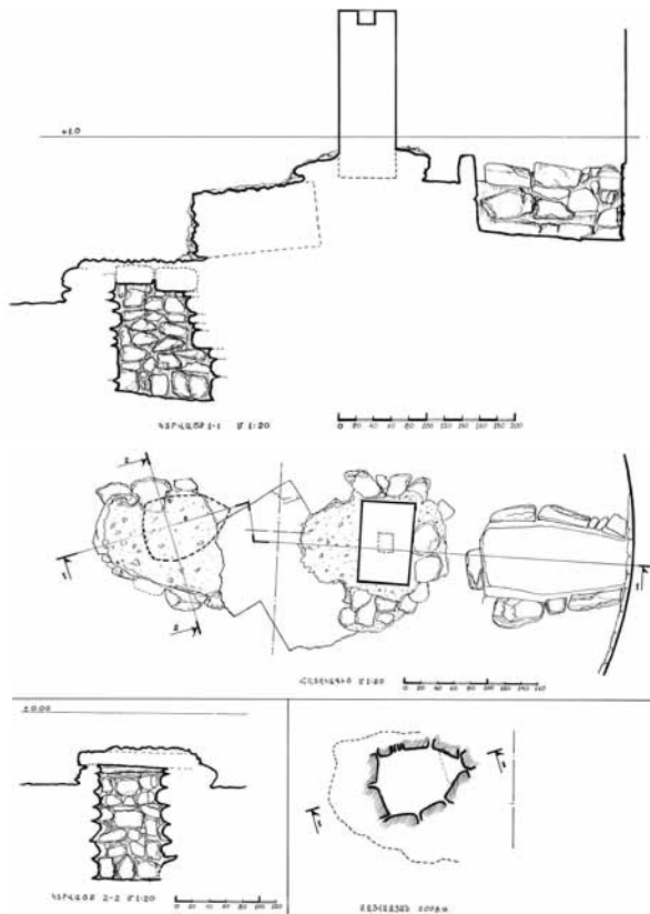
Խորանի կենտրոնական մասի կտրվածքը դեպի հյուսիս և հատակագիծը: Դամբարանի լայնական կտրվածքը և հատակագիծը (չափ.՝ Ս. Այվազյանի, 2008 թ.)
