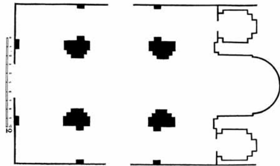
Մրեն. Կաթողիկե եկեղեցու առաջին չափագրությունը (հեղ.՝ հայր Ներսես Սարգսյան)
